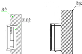
图3 暗装方式
