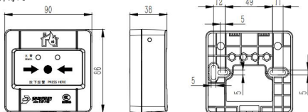
图 1 外形及安装尺寸图
