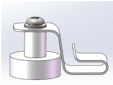
图 5 感温电缆在变压器上敷设示意图 磁吸安装专用夹具（JB-F4310-ZJ-02）
