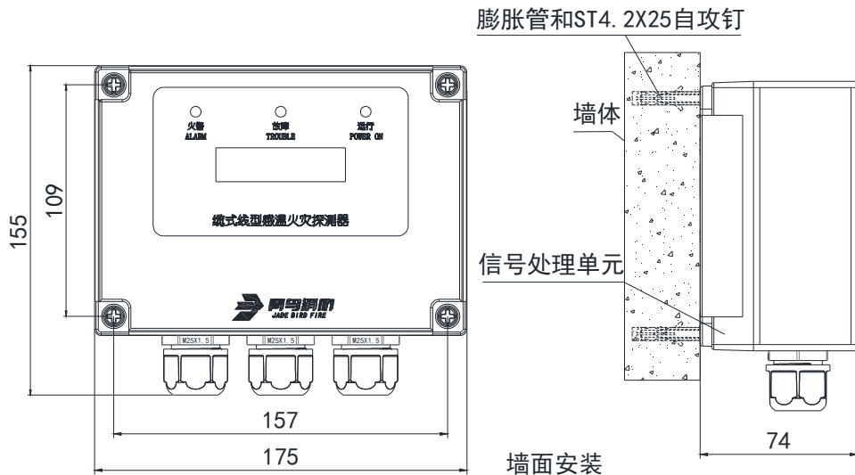
图 1 墙面安装示意图 (单位: mm)
