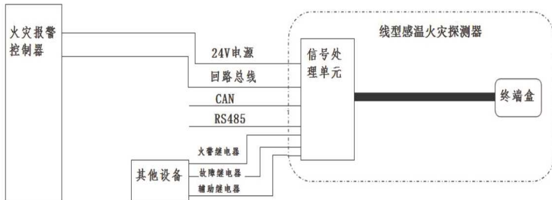
图 6 产品系统配接示意图
