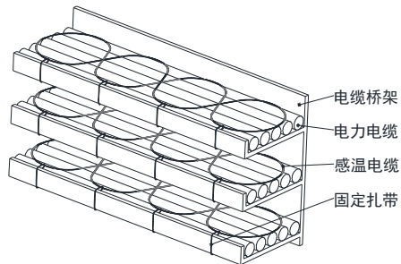
图 4 感温电缆敷设工程安装示意 2（线缆桥架应用为例） 电缆区域的火灾探测，感温电缆宜采用 S 型双绞接触式敷设。
