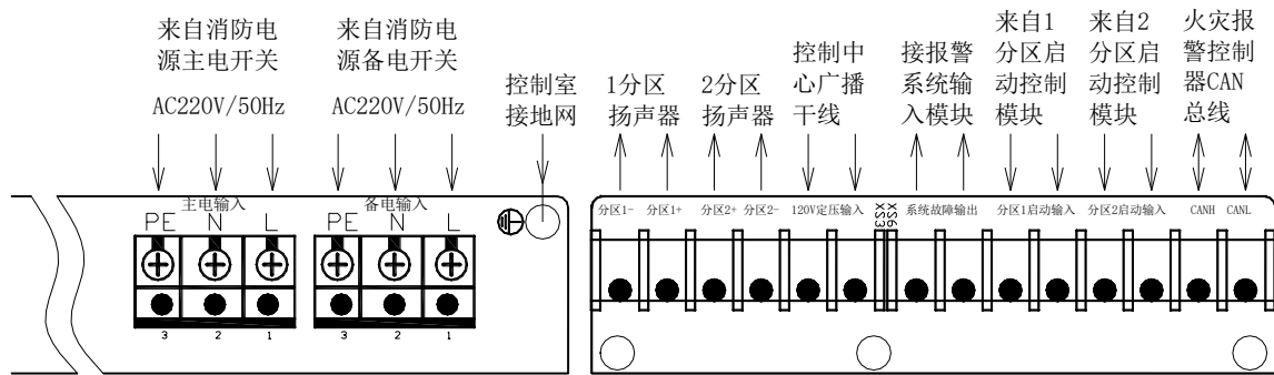
图4-1接线示意图
