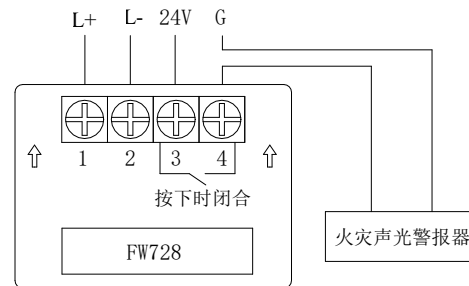
图 1. 端子接线图
