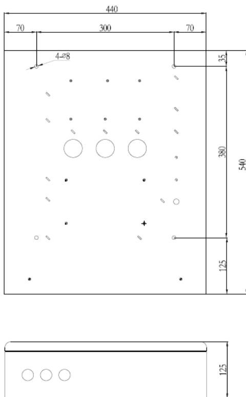
图2.3 监控设备安装尺寸图
