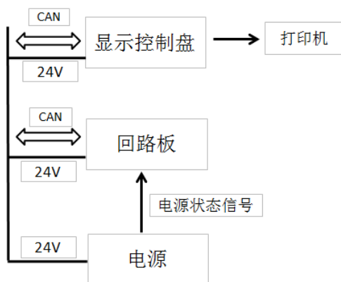
图2.1 JBF-61S30监控设备结构图
