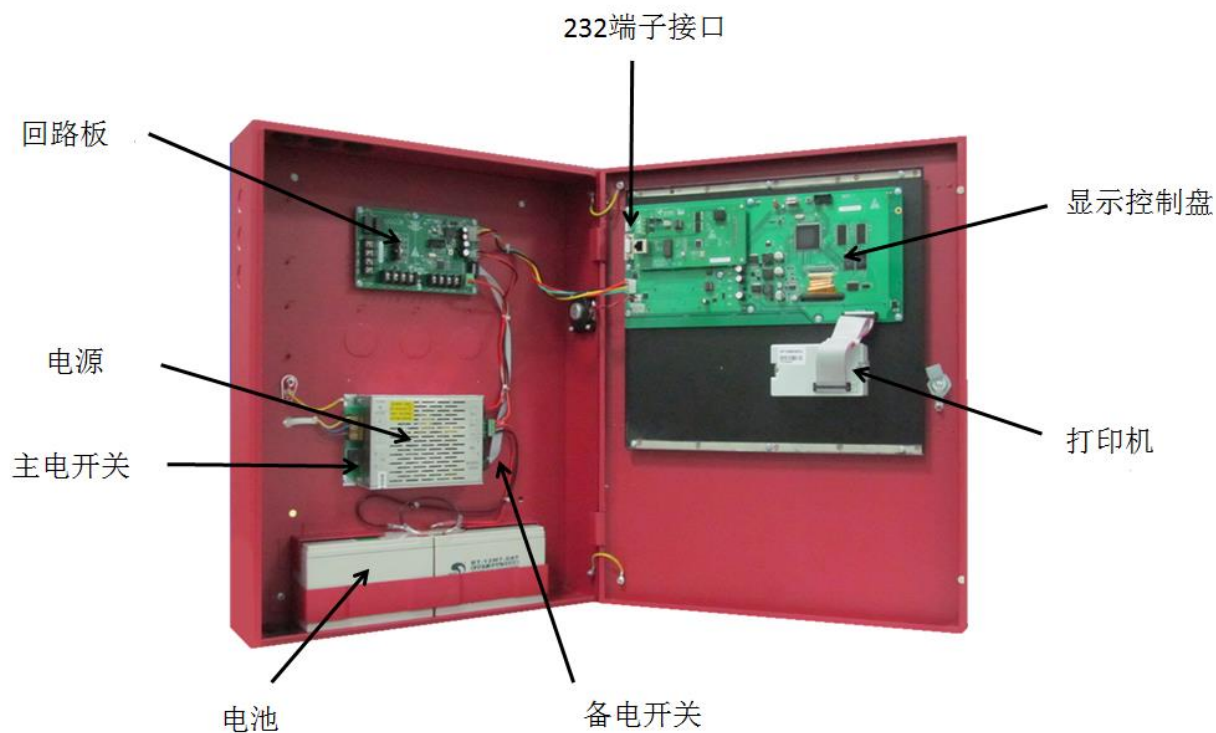
图2.5 监控设备内部结构图
