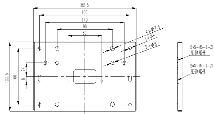
图 3 背板尺寸图
