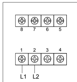
图 2 端子接线图
