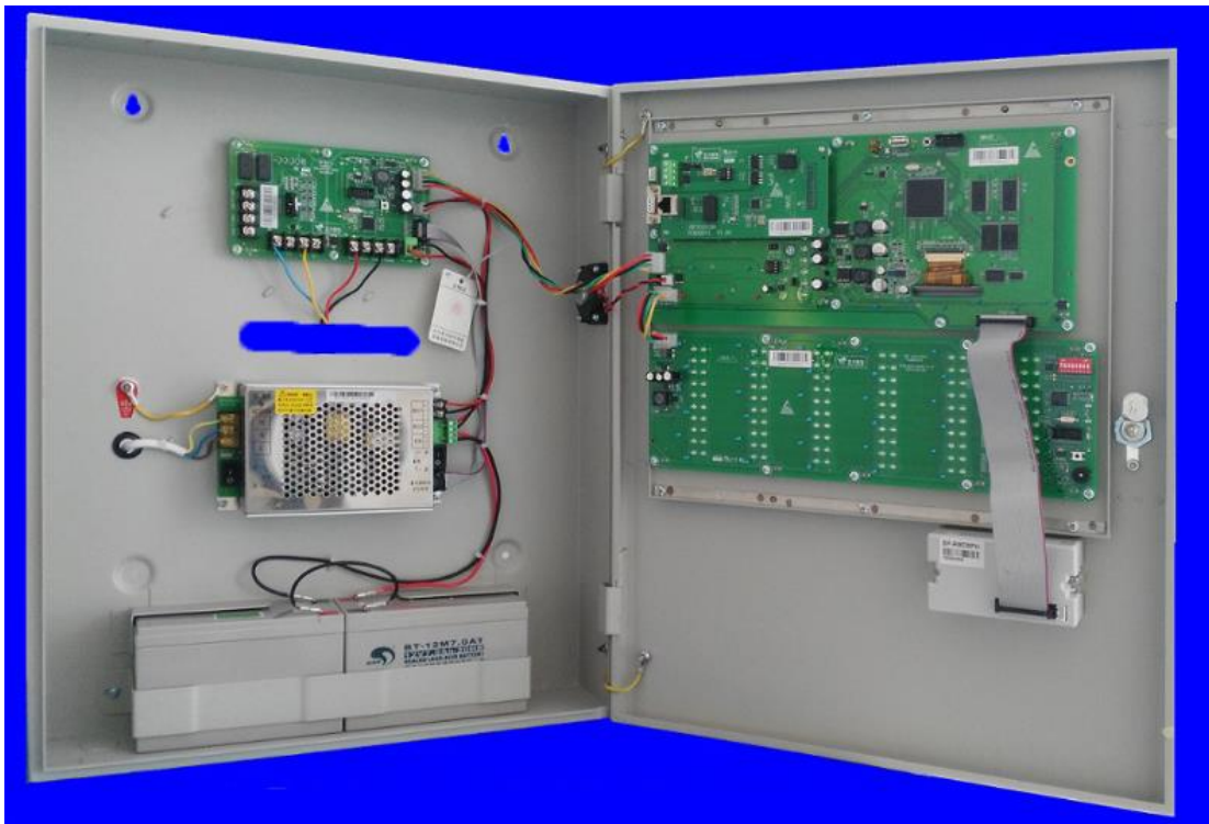
图4 JBF-61S20 壁挂机内部结构图
